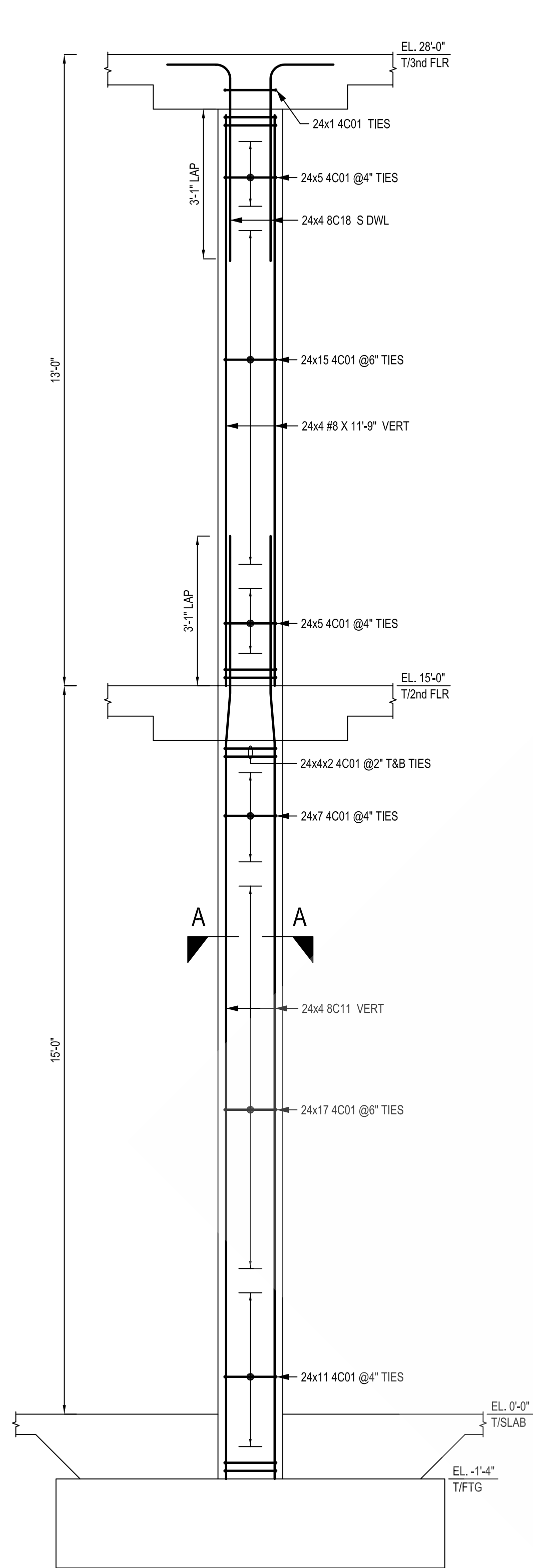
COLUMN - CC1 SCALE: 1/2"=1'-0" SDR: S1.6 (24 LOC)
