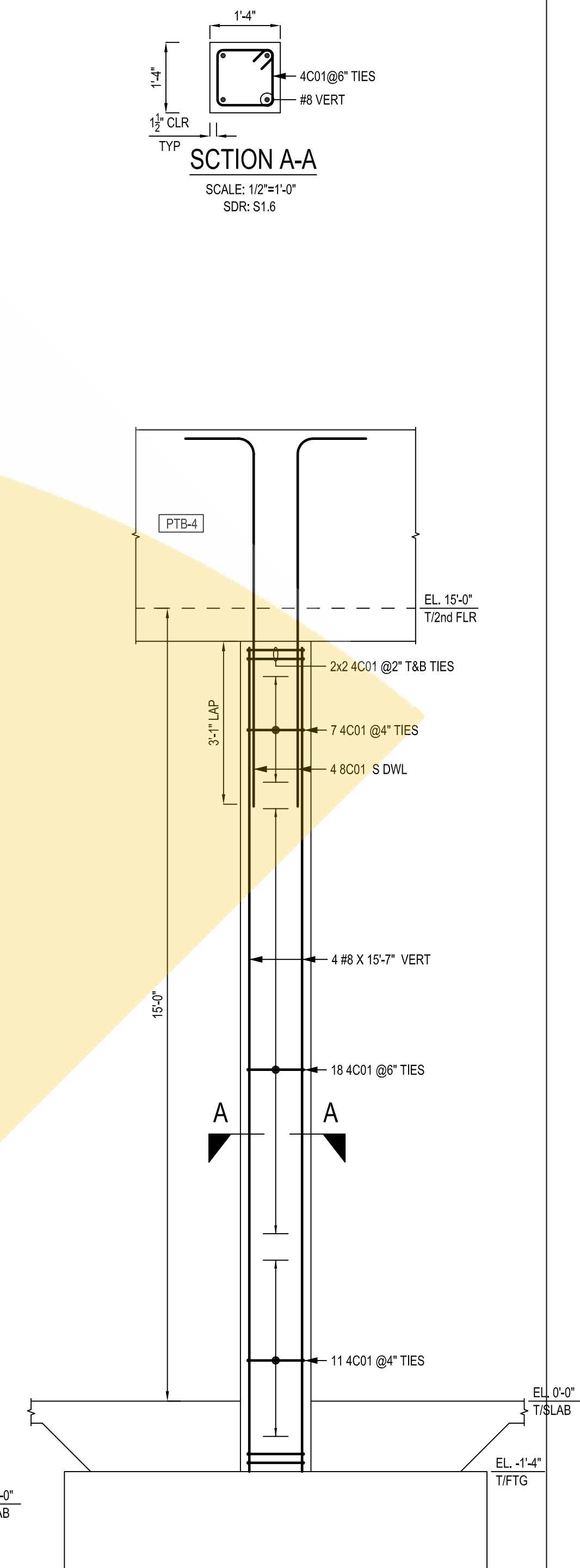
COLUMN - CC1d SCALE: 1/2"=1'-0" SDR: S1.6 (1 LOC)
