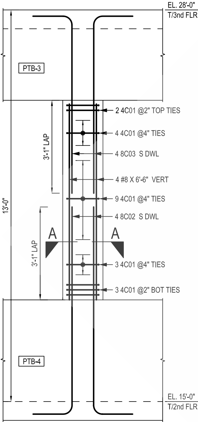
COLUMN - CC3 SCALE: 1/2"=1'-0" SDR: S1.6 (1 LOC)
